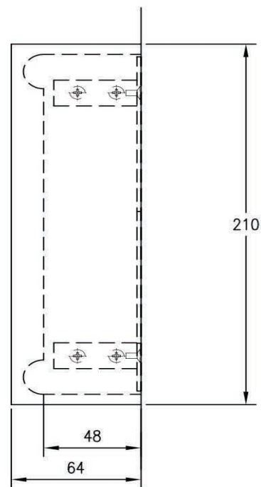
ELEVATION
