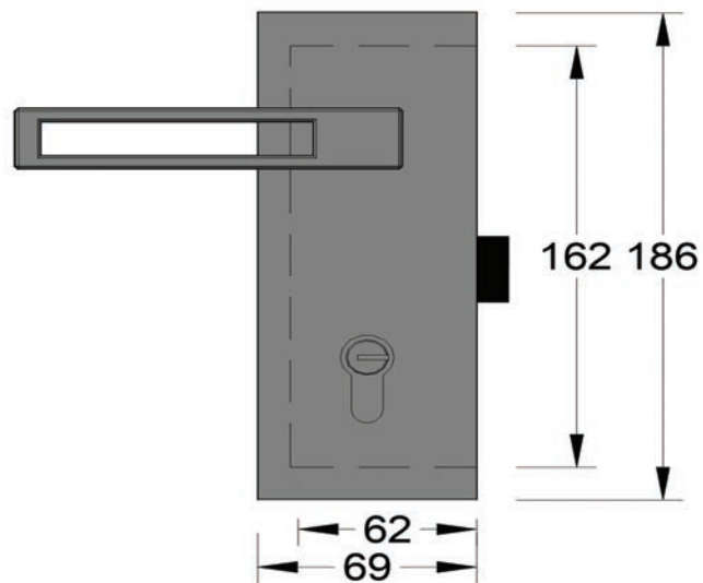
ELEVATION
