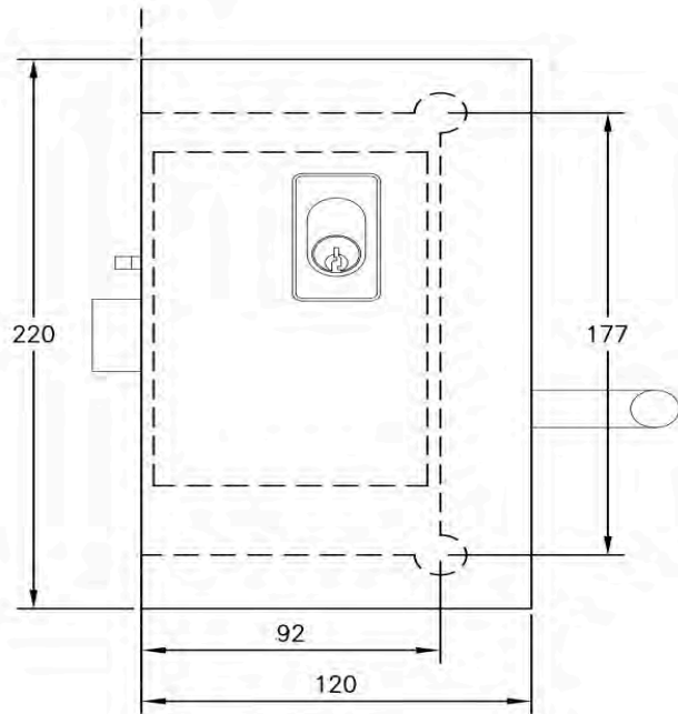
ELEVATION
