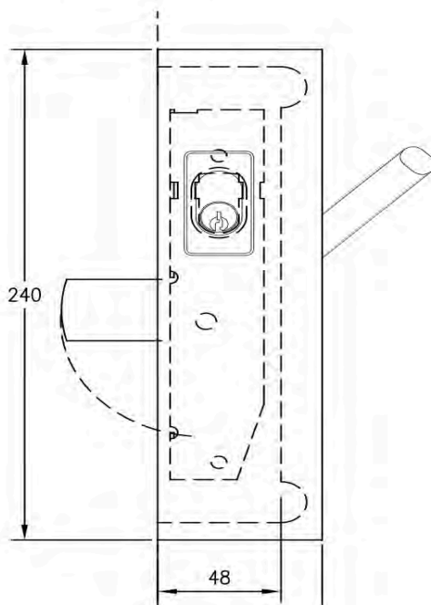
ELEVATION
