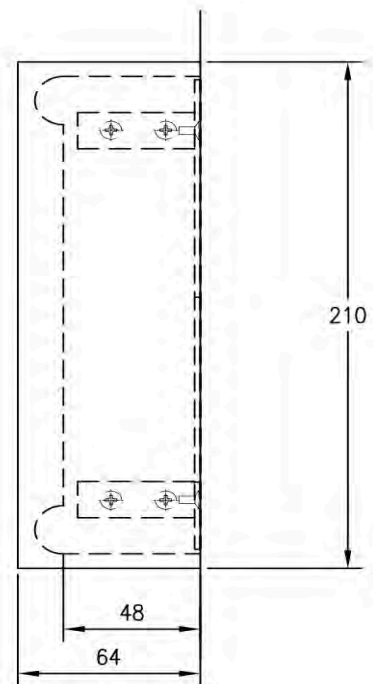
ELEVATION
