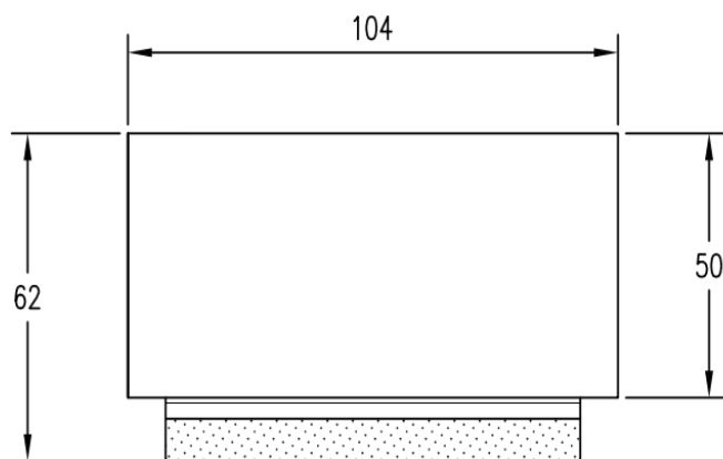
ELEVATION
